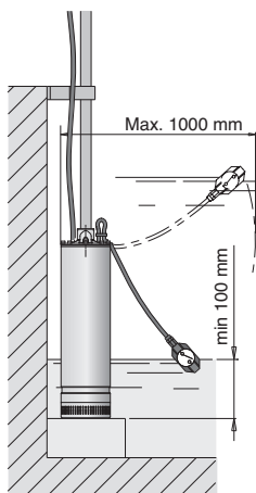
3.93.007/2 Exécution avec interrupteur à flotteur
