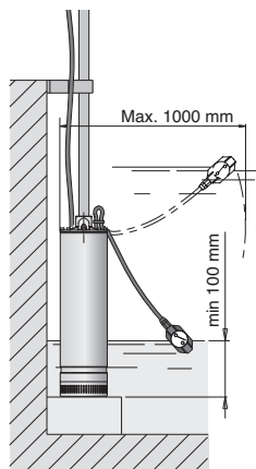
Ausführung mit Schwimmerschalter
