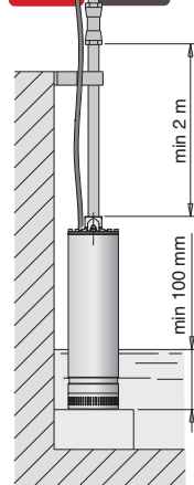
3.93.007/2 Οδηγίες για χρήση χωρίς φλοτέρ
