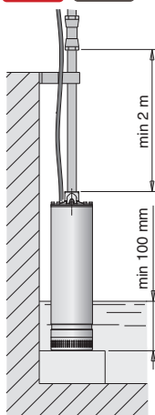
Esecuzione senza galleggiante
