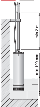
3.93.007/2 Exécution sans interrupteur à flotteur
