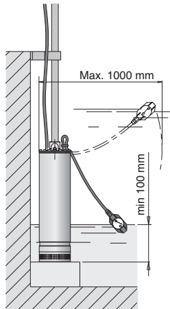
3.93.007/2 Οδηγίες για χρήση φλοτέρ
