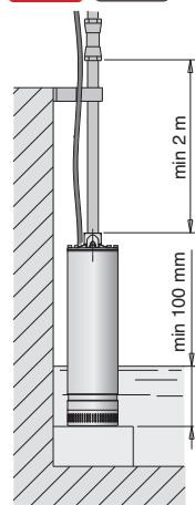
Pomp zonder vlotterschakelaar
